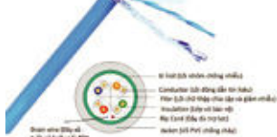
DÂY FTP
