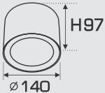
AFC 646D LED 12W Chất liệu: Thân đèn Sắt sơn tĩnh điện Tản nhiệt: Nhôm cao cấp Điện áp: 220V~50Hz Nguồn sáng: LED Ánh sáng: ● 3200K ○ 4200K ○ 6500K
