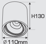
AFC 647D LED 7W Chất liệu: Thân đèn Sắt sơn tĩnh điện Tản nhiệt: Nhôm cao cấp Điện áp: 220V~50Hz Nguồn sáng: COB Góc chiếu: 24° Ánh sáng: ● 3200K ○ 4200K ○ 6500K
