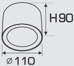
AFC 646D LED 9W - 9W ●○○ 3 chế độ sáng Chất liệu: Thân đèn Sắt sơn tĩnh điện Tản nhiệt: Nhôm cao cấp Điện áp: 220V~50Hz Nguồn sáng: LED Ánh sáng: ● 3200K ○ 4200K ○ 6500K
