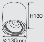
AFC 647D LED 12W Chất liệu: Thân đèn Sắt sơn tĩnh điện Tản nhiệt: Nhôm cao cấp Điện áp: 220V~50Hz Nguồn sáng: COB Góc chiếu: 24° Ánh sáng: ● 3200K ○ 4200K ○ 6500K
