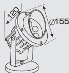
NGŨI CỎ LED 12W
