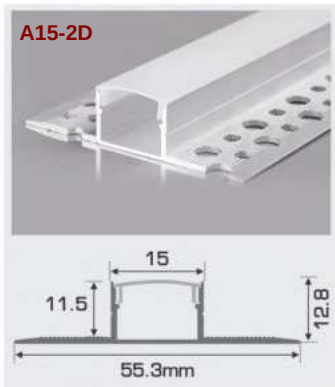
A15 - 2 D W55.3 x H12.8mm 1.5m 234.000 Nhôm định hình + Chụp nhựa PC
