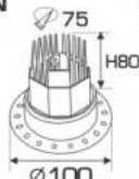
AFC 795 T - 9W ÂM VIỀN 438.000
