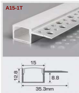
A15 - 1 T W35.3 x H12.8mm 1.5m 204.000 Nhôm định hình + Chụp nhựa PC
