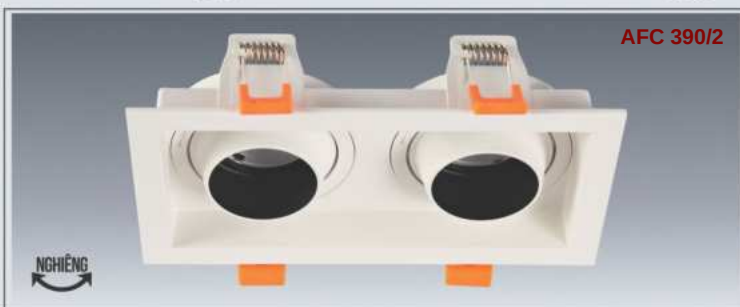
AFC 390/2 - MR16 (Không Bóng) 608.000 Thân đèn: Hợp kim nhôm cao cấp Khoét lỗ: 80 x 160mm
