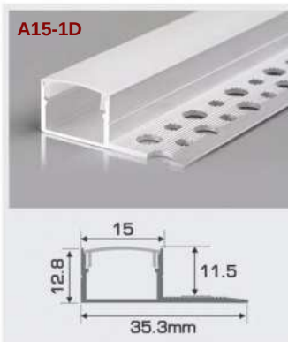
A15 - 1 D W35.3 x H12.8mm 1.5m 204.000 Nhôm định hình + Chụp nhựa PC
