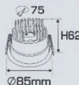
AFC 736 D LED 9W 394.000
