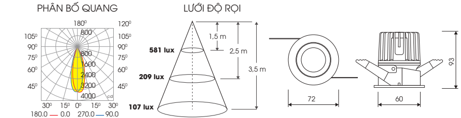
AT22 60/7W
