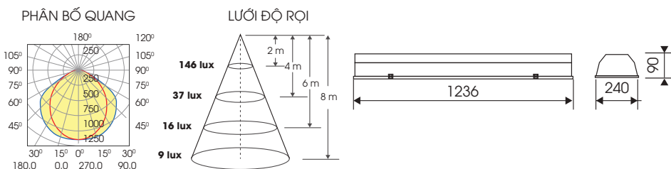
T8 CSLH/20Wx1
