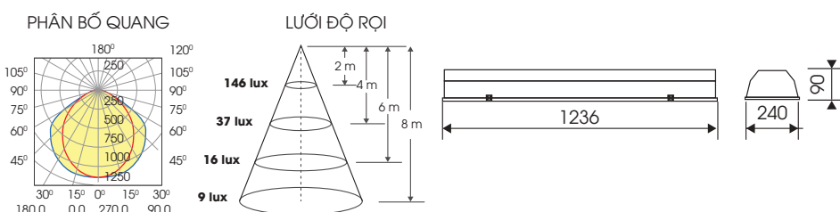
T8 CSLH/20Wx2
