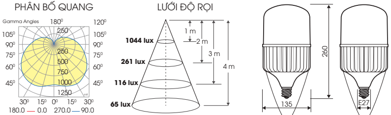
TR135ND/80W.H
