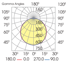
LN26 300/25W
