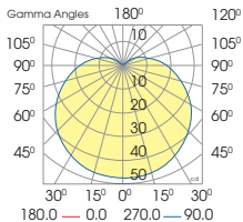
A55N4/5W.H
