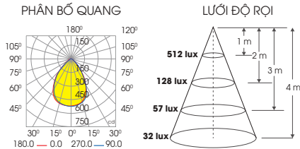
NT01 110/15W
