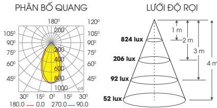
NT01 110/12W
