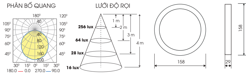
LN09 170/15W
